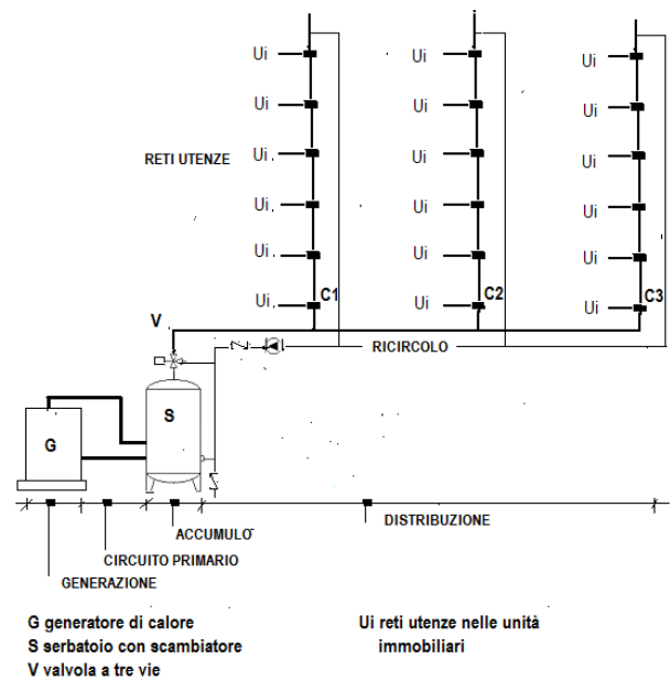
Figura 7.3 – Schema rete di distribuzione (Fonte: UNI TS-11300-2:2014)
